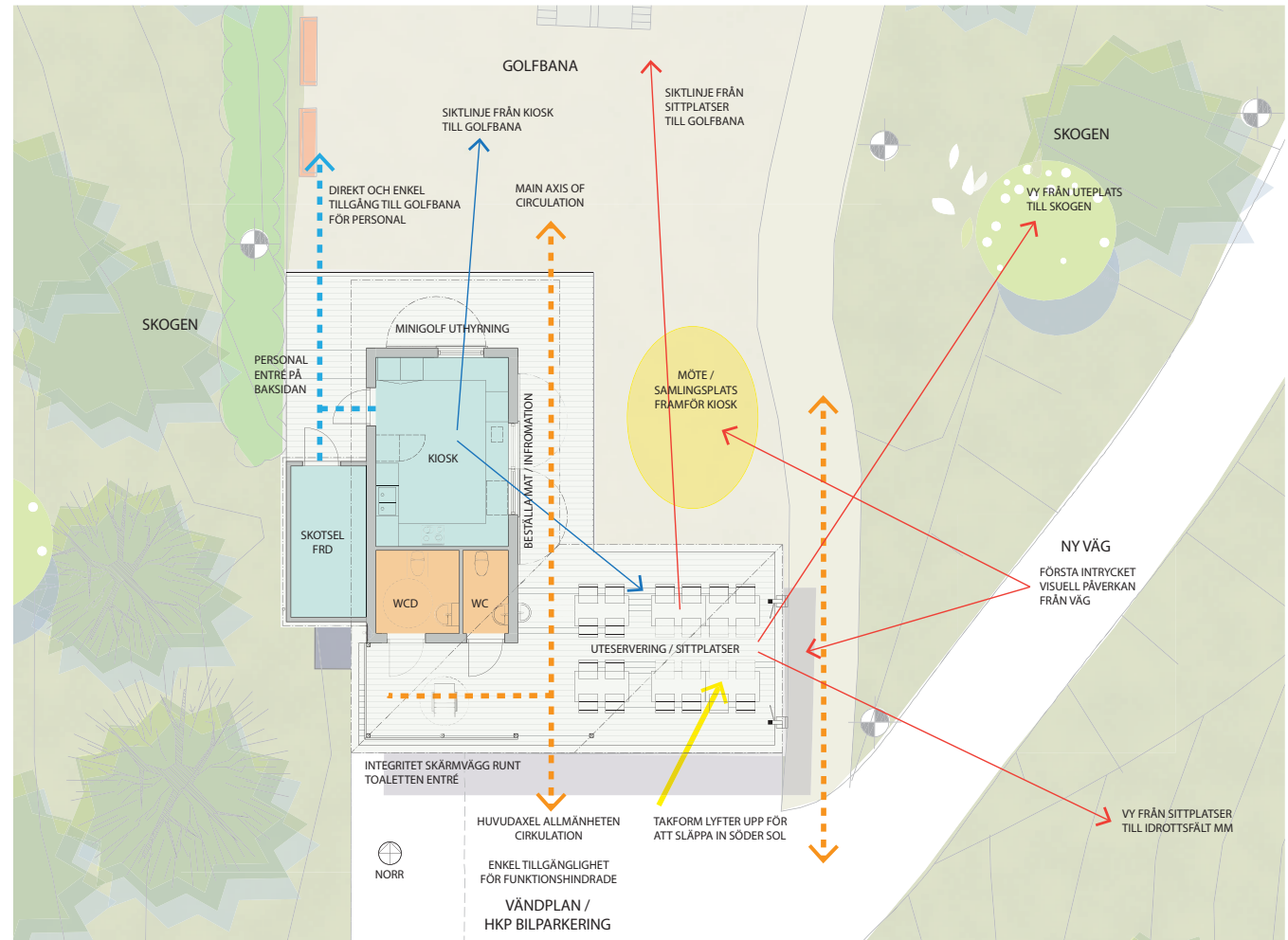
PLAN KLUBBHUS/KIOSK
